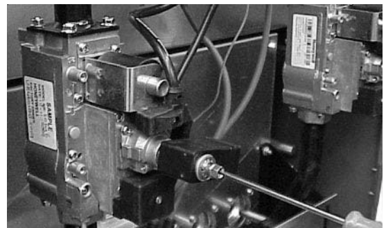
Reglaje tornillo de ajuste para nivel de presión mínimo
